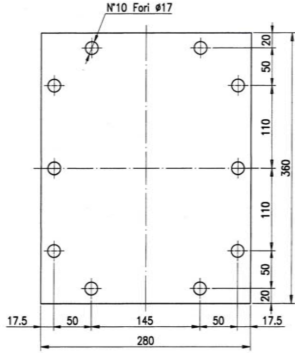
PIASTRA BASE · PLATE · PLAQUE · CHAPA · PLATTE: min. 15mm
